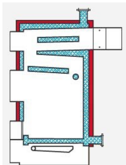
Innenaufbau Schema
